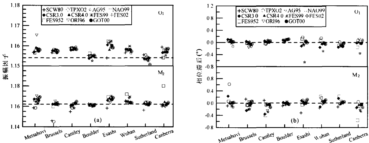
图 4 几个 GGP 台站主波 O_1 和 M_2 的海潮负荷改正后的振幅因子(a)和相位滞后(b)
