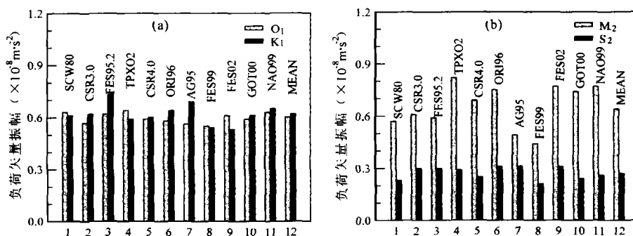
图 1 周日频段(a)和半日频段(b)内主波重力负荷矢量振幅
