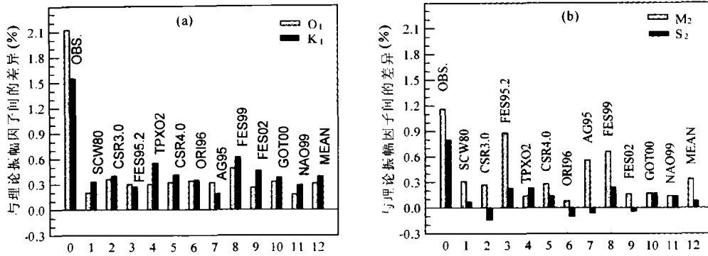
图 3 周日频段(a)和半日频段(b)内海潮负荷改正前后主波振幅因子与理论值间的差异
